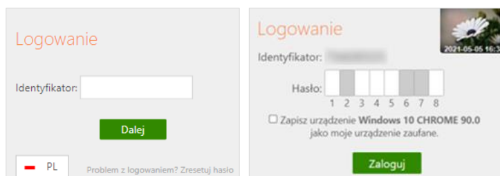
Rys.1 Okna „Logowanie”.
